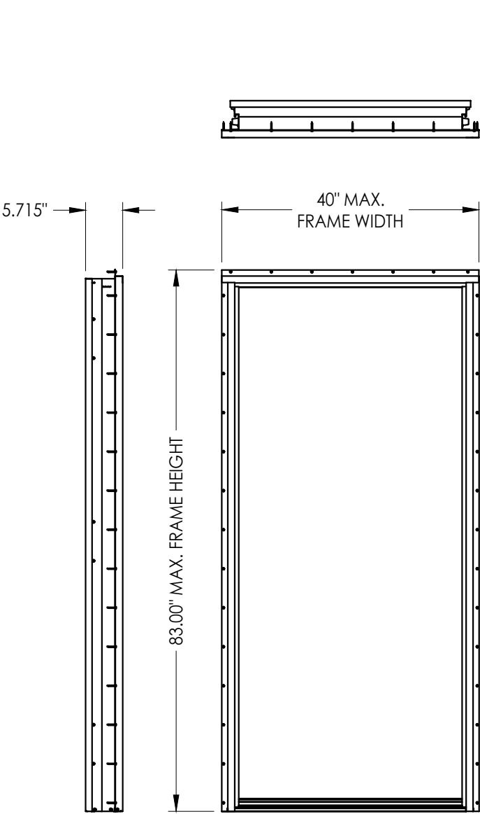
FRAME ELEVATION
